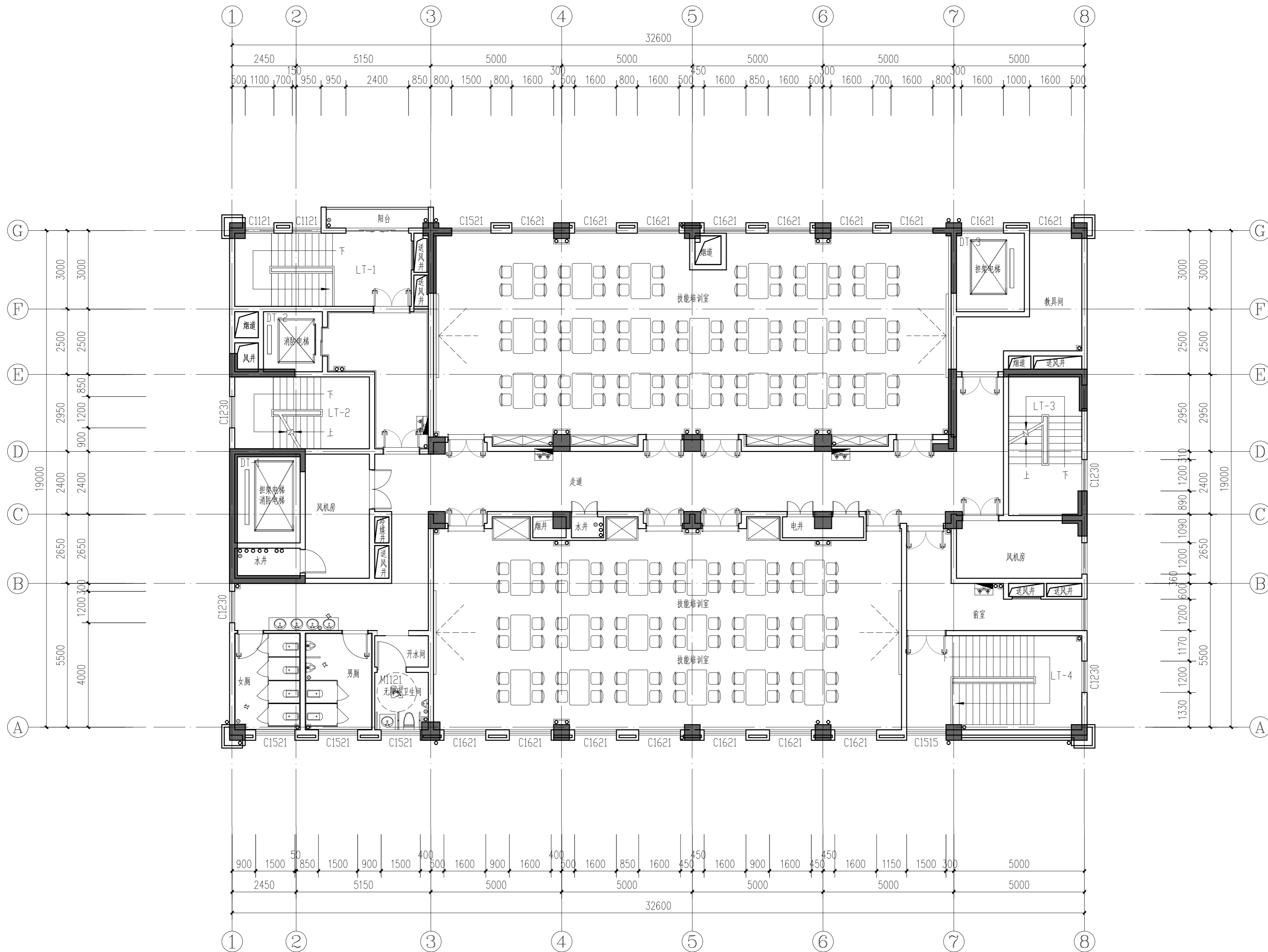
五层平面图 1:100
