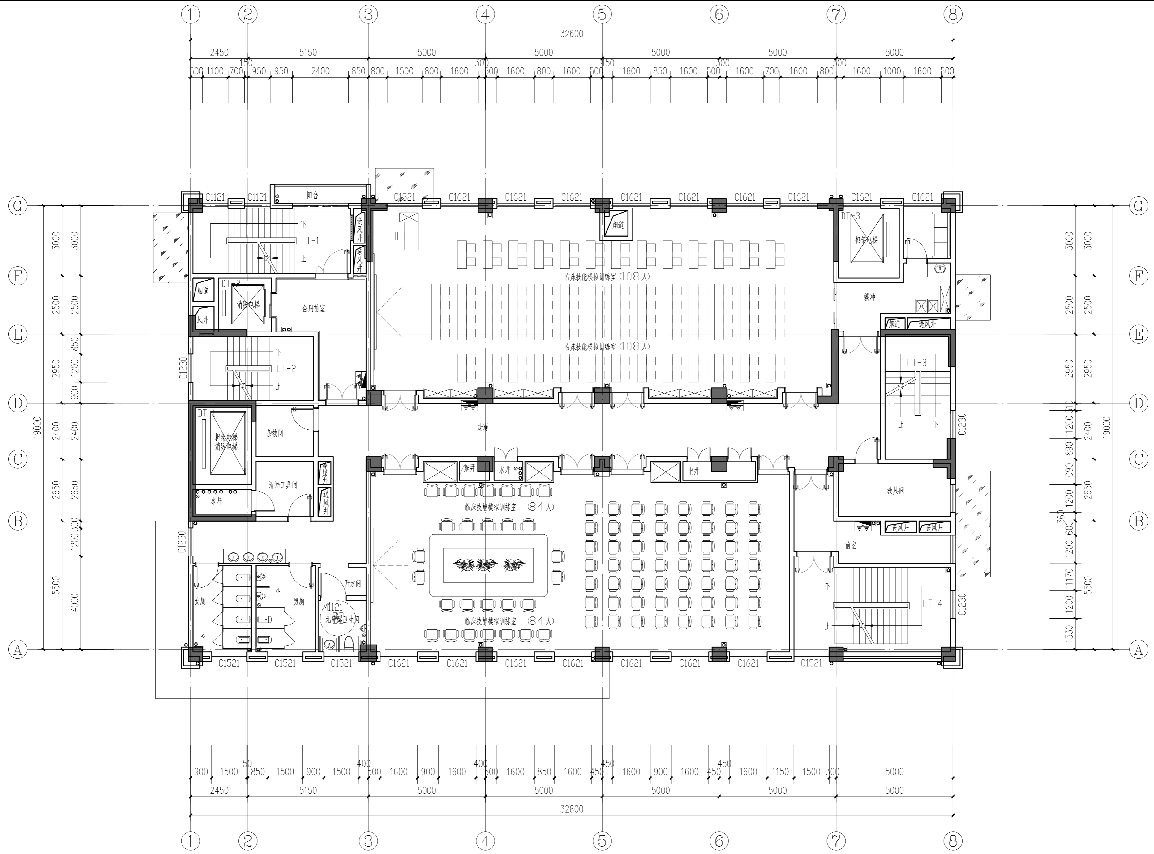
三层平面图 1:100
